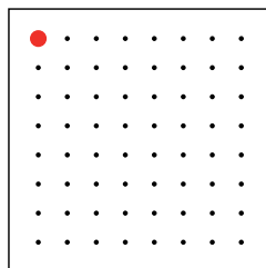
тахир шугам
