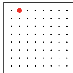
дөрвөлжин
