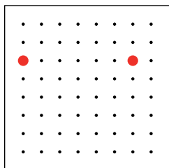
хэрчим
